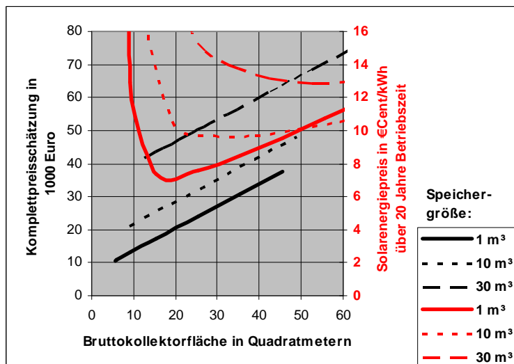
Bild 6 Die Komplettkosten der Solar- und Kombispeicheranlage (schwarze Linien) und solare Energieentstehungskosten (rote Linien) in Abhängigkeit von der Kollektorfläche für verschiedene Speichergrößen
